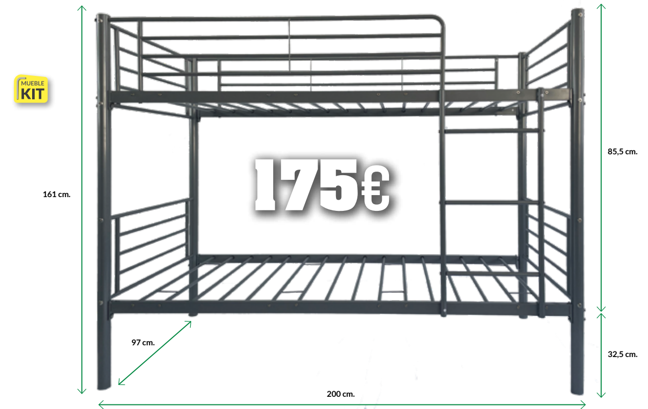
38. Litera metálica pintada con pintura electrostática color gris. Somieres incluidos para colchones de 90x190 cm.
